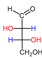
D-threose
